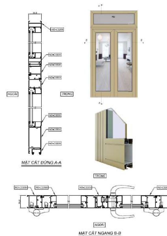
CỬA ĐI VÀ CỔ ĐỊNH HỆ XF55
