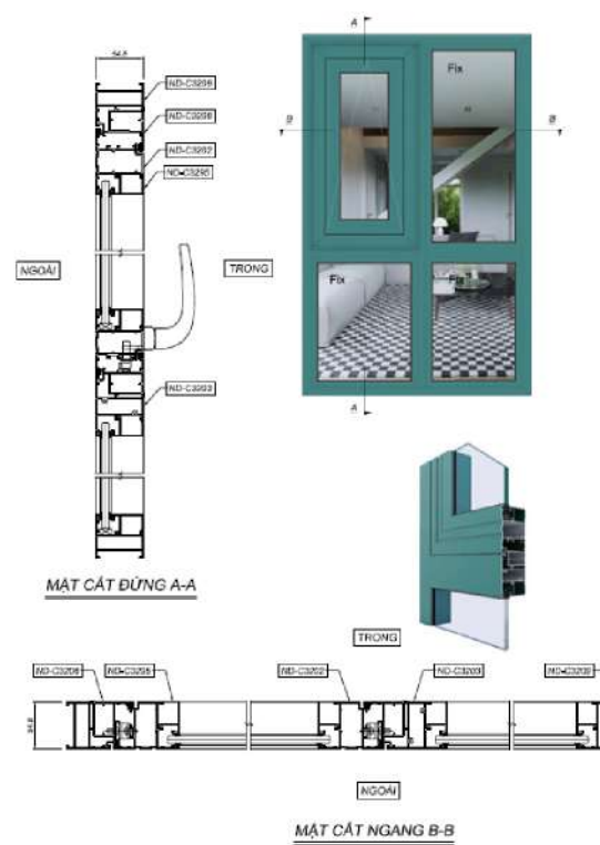
CỬA SỔ MỞ LẬT HỆ XF55
