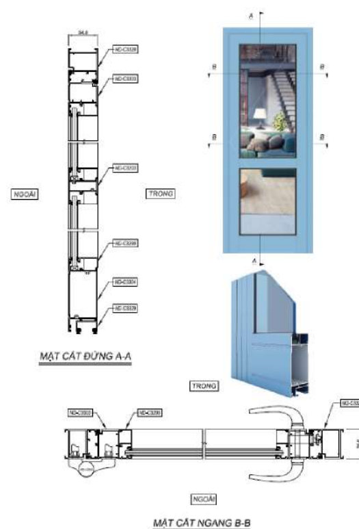
CỬA ĐI HỆ XF55
