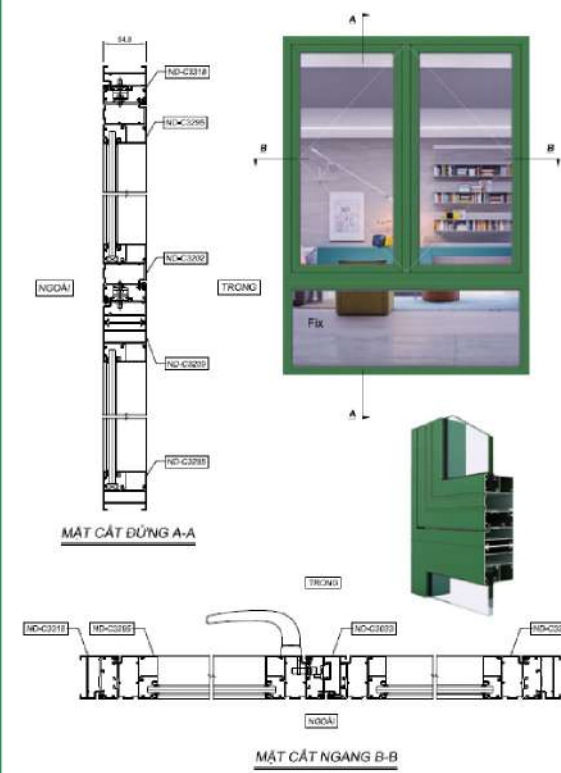
CỬA SỔ MỞ QUAY HỆ XF55
